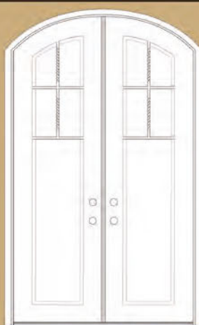
Door Unit: 207296 Scroll Design: 067296B
